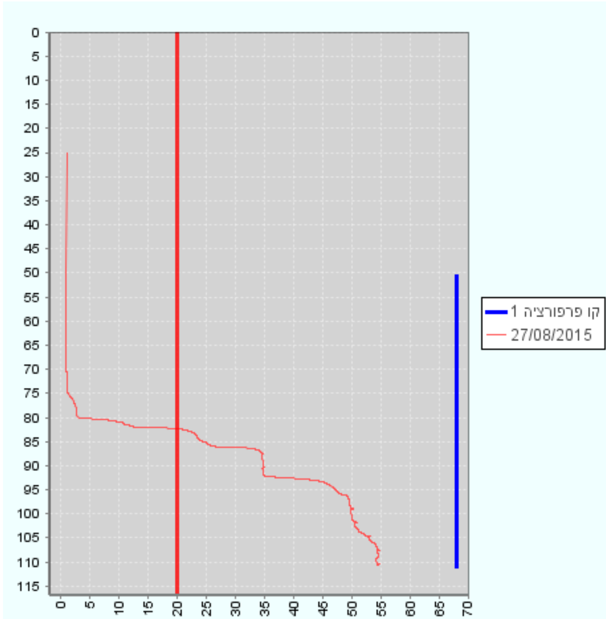
פרופיל מוליכות חשמלית של קידוח מח 104 ת2 (11510504). ציר ה-Y, עומק (מ'), ציר ה-X, מוליכות חשמלית mS/cm.
